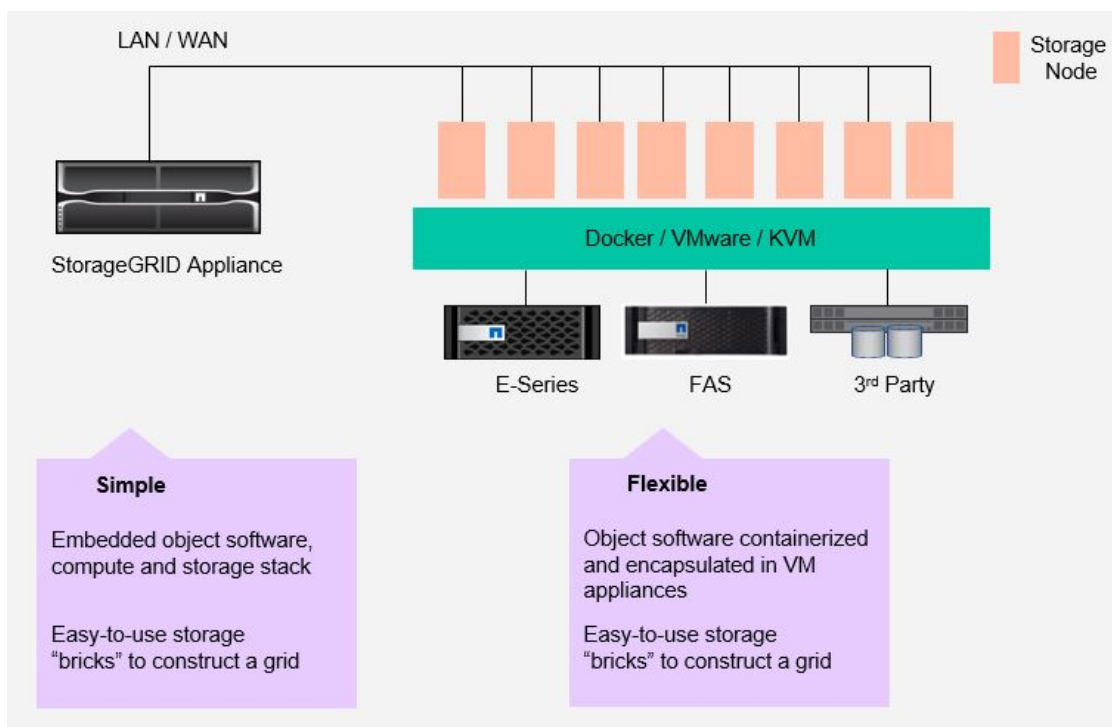
Figure 4 : Des appliances de nœuds de stockage physiques et virtuelles peuvent être déployées dans la même grille.
